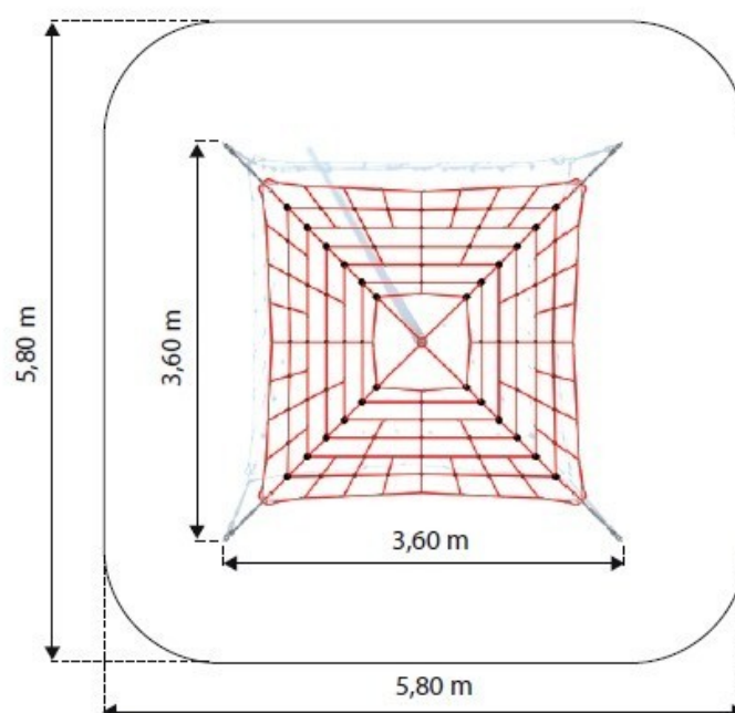
Rys. 1. Wymiary urządzenia i strefy bezpieczeństwa
