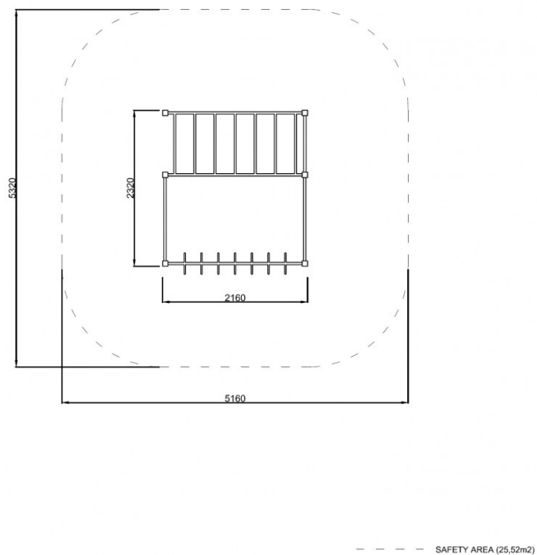
Rys. 1. Wymiary urządzenia i strefy bezpieczeństwa
