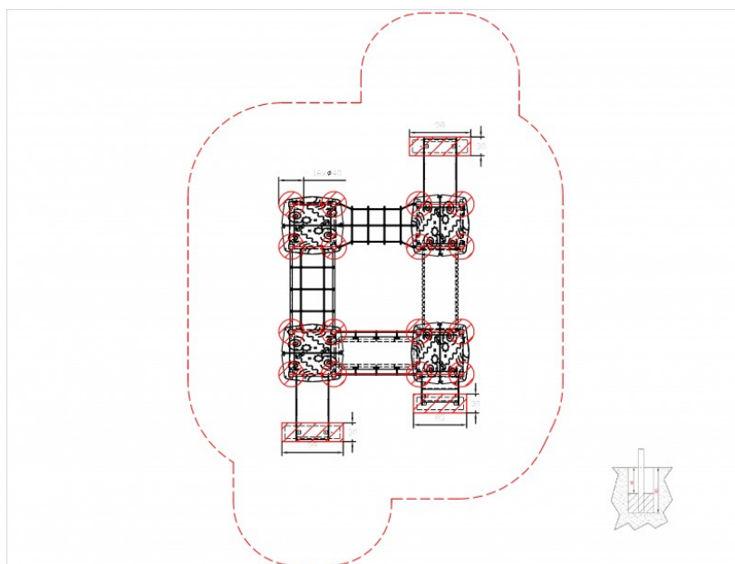
Rys. 2. Fundamenty
