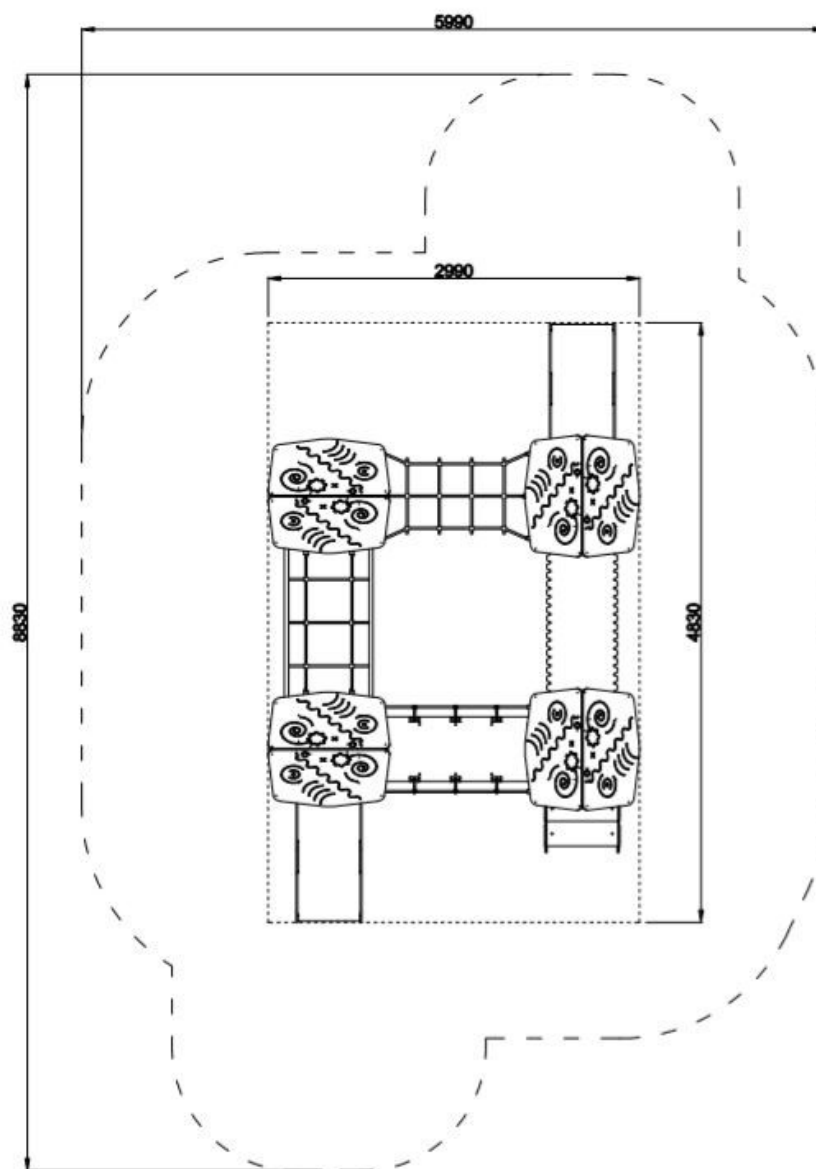
Rys. 1. Wymiary urządzenia i strefy bezpieczeństwa
