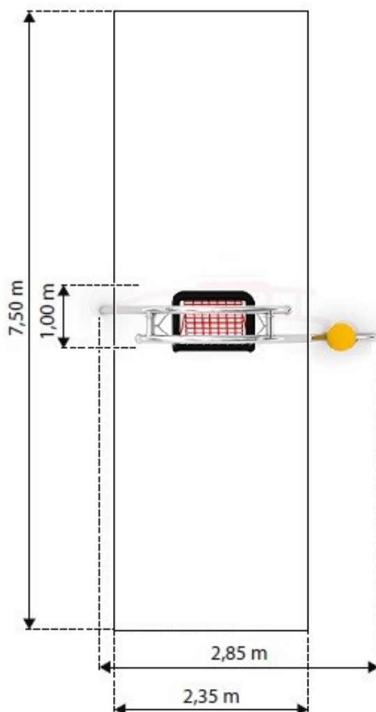
Załącznik 1. Wymiary urządzenia i strefy bezpieczeństwa
